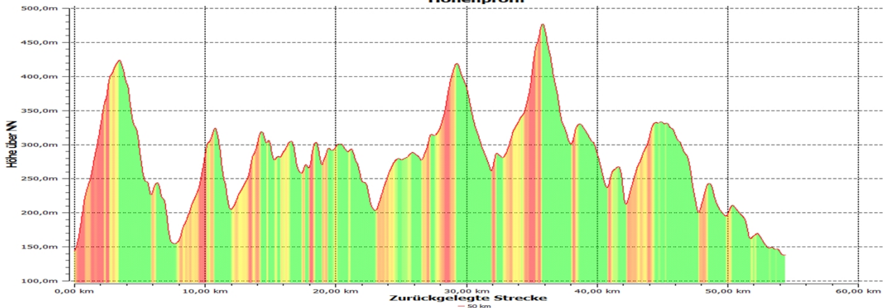
Höhenprofil
